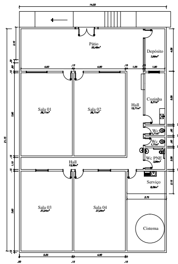
1 PLANTA BAIXA SITUAÇÃO ATUAL ESCALA 1:100
