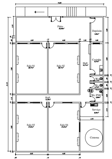
3 PLANTA BAIXA FINAL ESCALA 1:100
