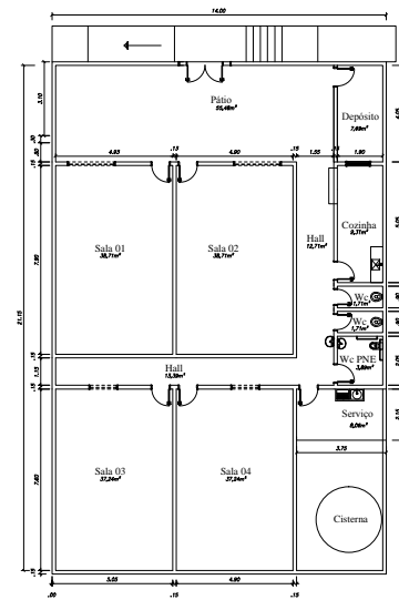
2 PLANTA BAIXA REFORMA ESCALA 1:100
